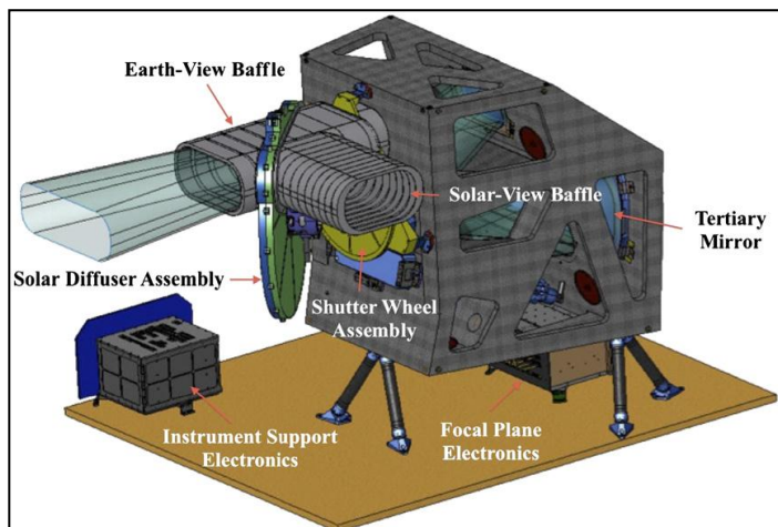
Figure 2-2. OLI Instrument
